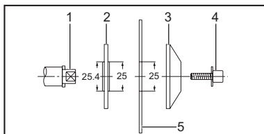
► 1. Eje de montaje 2. Brida interior 3. Brida exterior 4. Tornillo hexagonal 5. Disco
